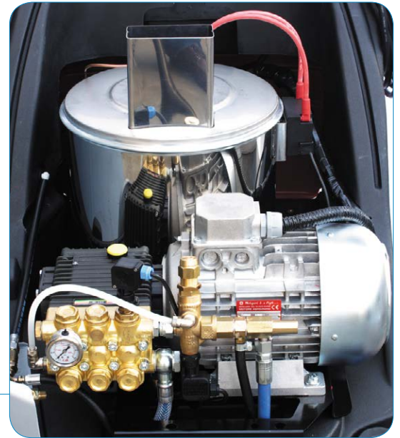
Geschickte Struktur mit bequemem Zugang zu Innenteilen bei Wartung.
